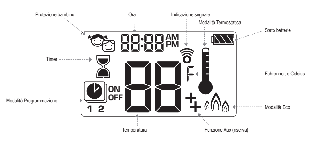
Fig. 21: Display a 8 caratteri
