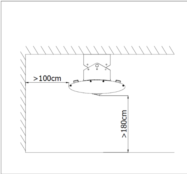
Plafond montage:
