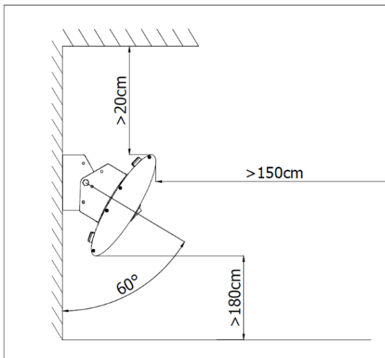
Montage mural :
