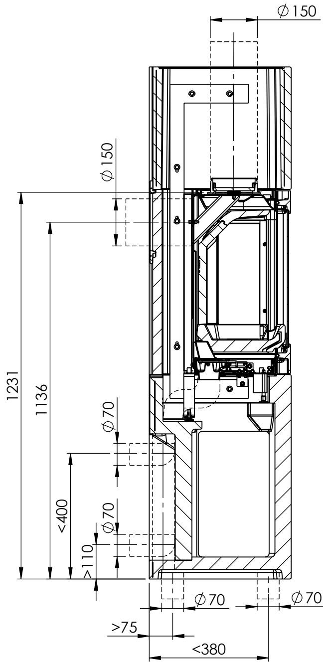
SECTION A-A
