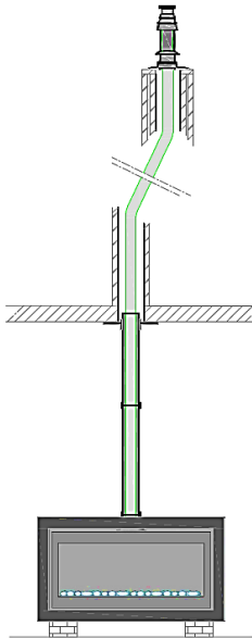
Schouwkanaal als luchttoevoer Renovatiekitt (C 91 )
