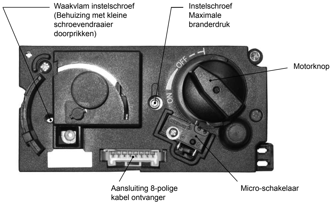
Figuur 17: Gasregelblok - Voorzijde
