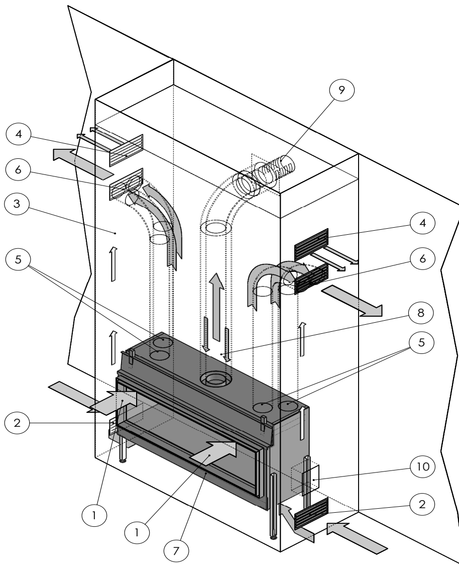
Figuur 13: Toestel ingebouwd in geventileerde schouw Horizontale uitmondning van de rookgasafvoer/verbrandingslucht- toevoer via de muur.
