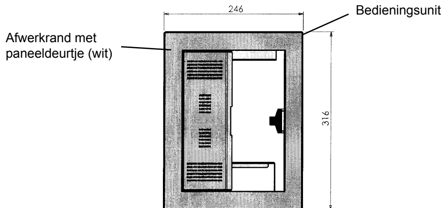
Figuur 15: Bedieningsunit
