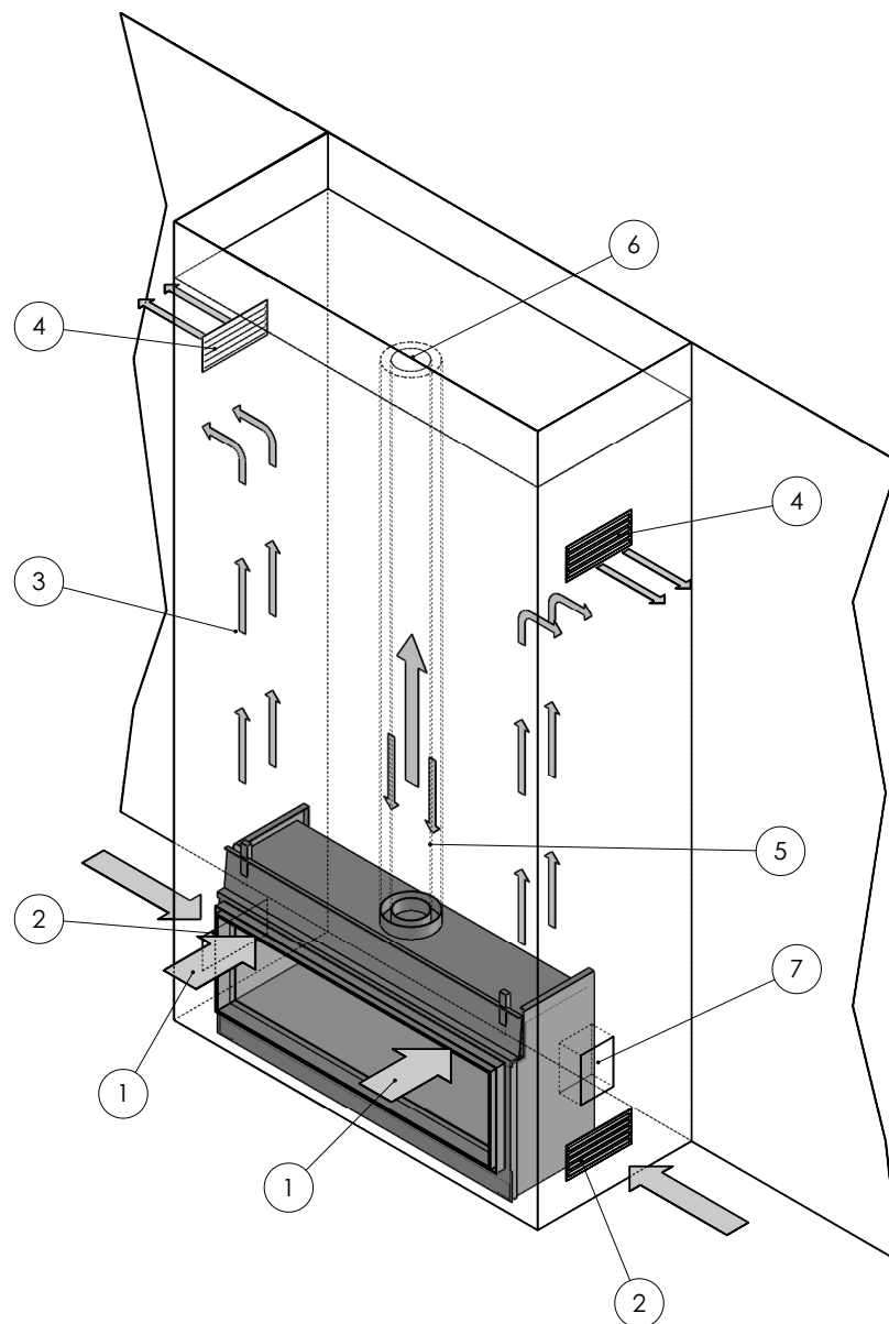
Figuur 14: Toestel ingebouwd in geventileerde schouw Verticale uitmonding van de rookgasafvoer/verbrandingslucht- toevoer via het dak. Toepassing zonder convectiepakket
