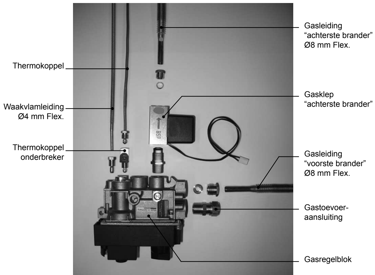
Figuur 16: Gasregelblok en gasklep: Gas en thermokoppel aansluitingen
