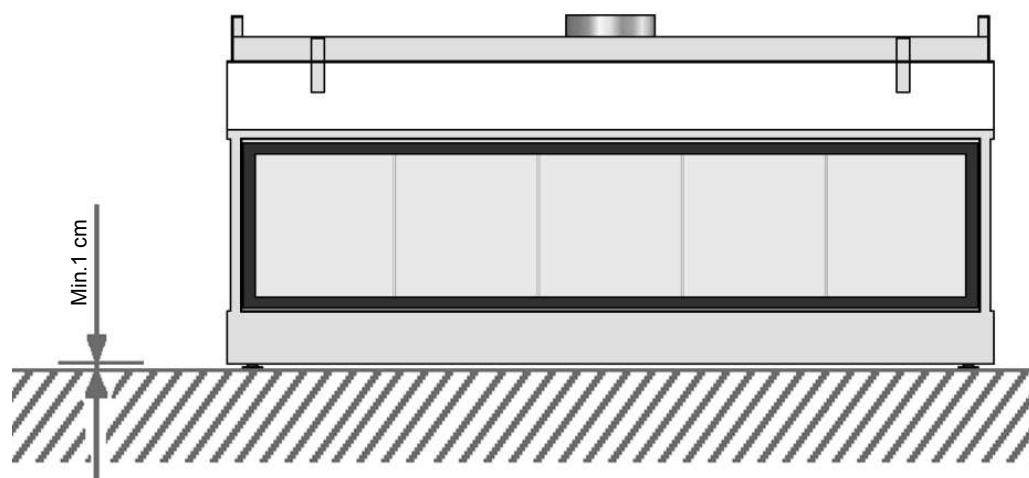
Figuur 12: Minimaal 1 cm ruimte tussen onderzijde toestel en vloer
