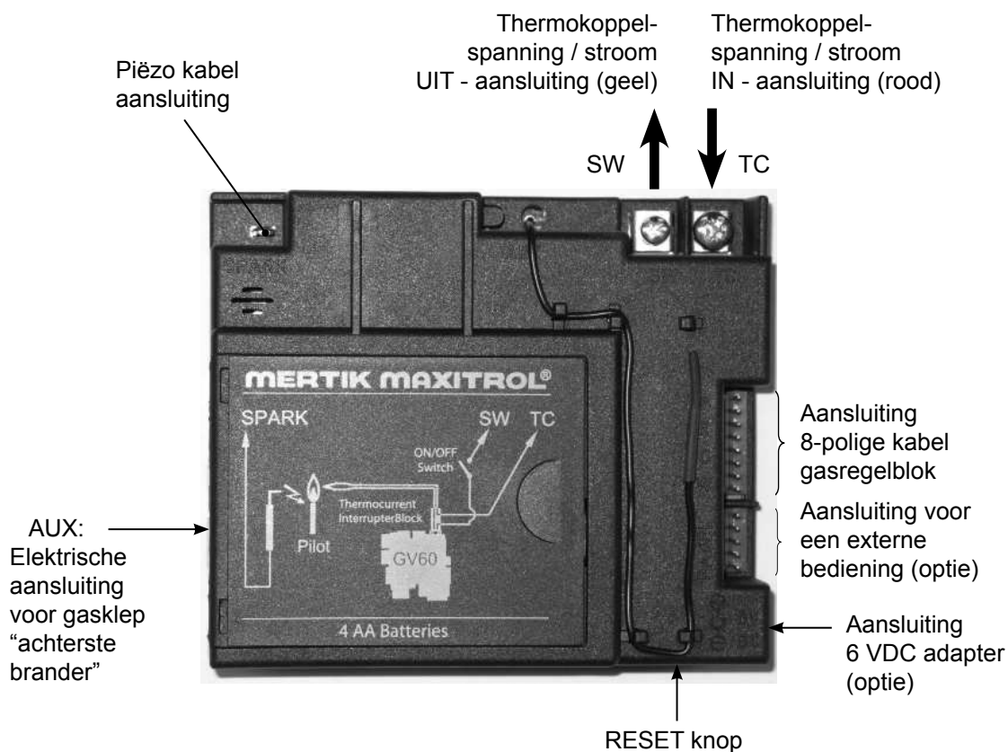
Figuur 19: Ontvanger - Bovenzijde
